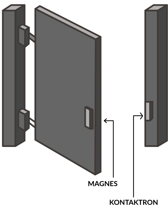
6. Schemat montażowy: czujnik kontaktronowy
