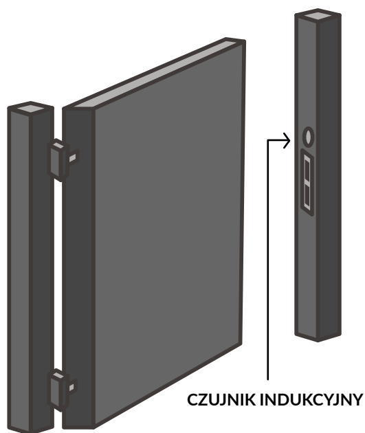
7. Schemat montażowy: czujnik indukcyjny
